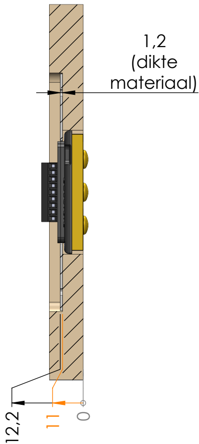
SECTION A-A
